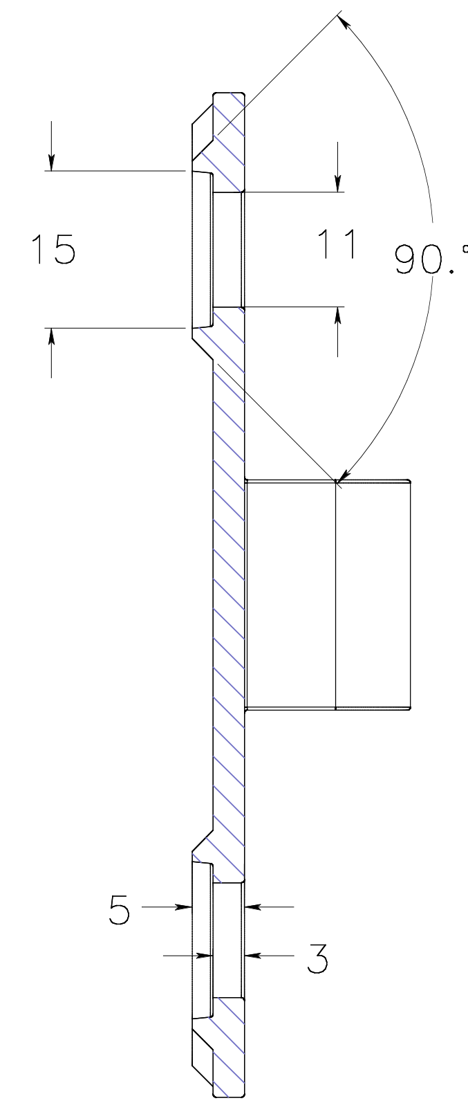
section DD
